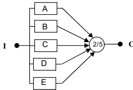
Figure 16 – 2 sur 5 système non identique
