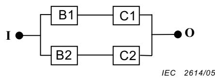
Figure 11 – Représentation de la Figure 8, quand l'entité A est défective
