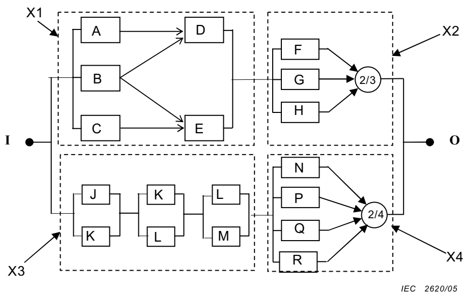
Figure 17 – Illustration de groupements de blocs avant réduction
